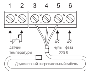
Схема подключения двухжильной нагревательной секции ProfiRoll
