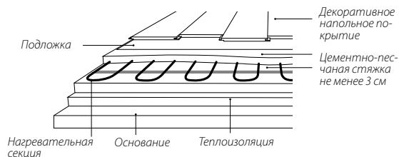
Схема укладки под ламинат, линолеум или ковровый в холодных помещениях
