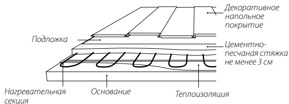
Схема укладки под ламинат, линолеум или ковровлин
